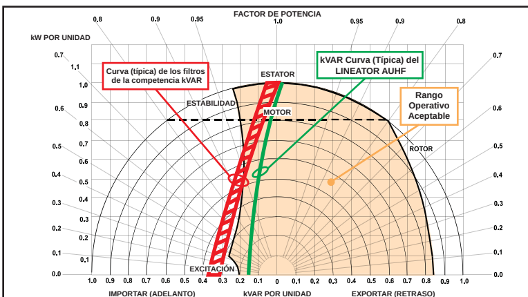
Curva de capacidad del generador de potencia reactiva
